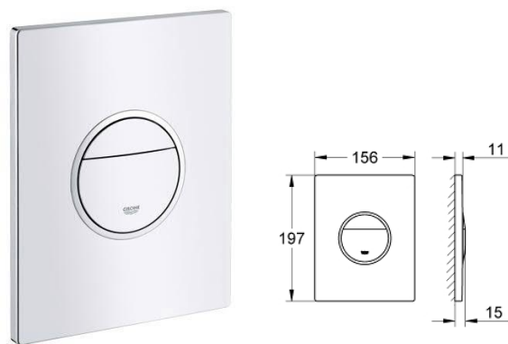
38 766 000 GROHE Ondus Wall Plate
