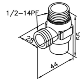
6790-TA-80CR Diverter
