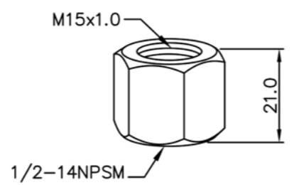
6771-W7-80CR Connector
