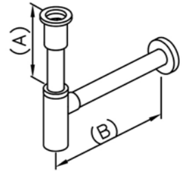
T-Trap 6502-TT-80CP A:170 B:340(mm) 6502-TT-81CP A:170 B:465(mm)
