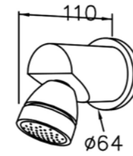
6880-AH-80CP Showerhead
