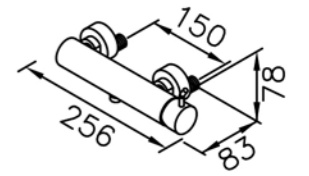
6768-93-80CP Shower Mixer Body
