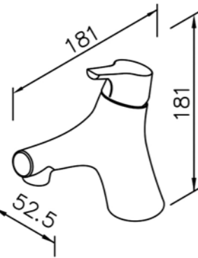
6927-90-80CP Basin Faucet
