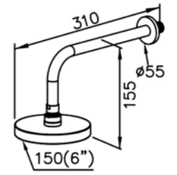
6771-AH-80CP 6" Showerhead
