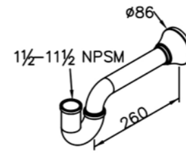
P-Trap 6122-A3-80CP 1 1/2" 6122-B3-80CP 1 1/4"
