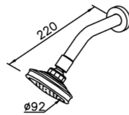
6803-AH-80CP Showerhead
