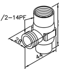
6790-TB-80CR Diverter
