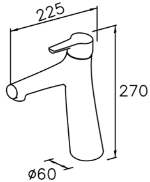
7927-90-80CP Basin Faucet
