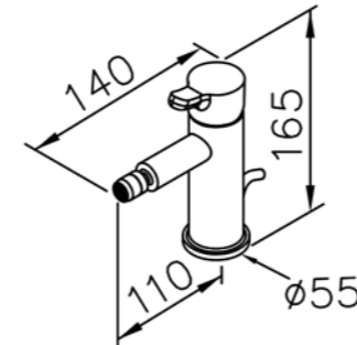
6766-99-81CP Bidet Mixer
