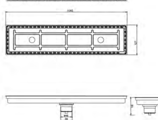
0306-54-79S1 Floor Drain SUS 304
